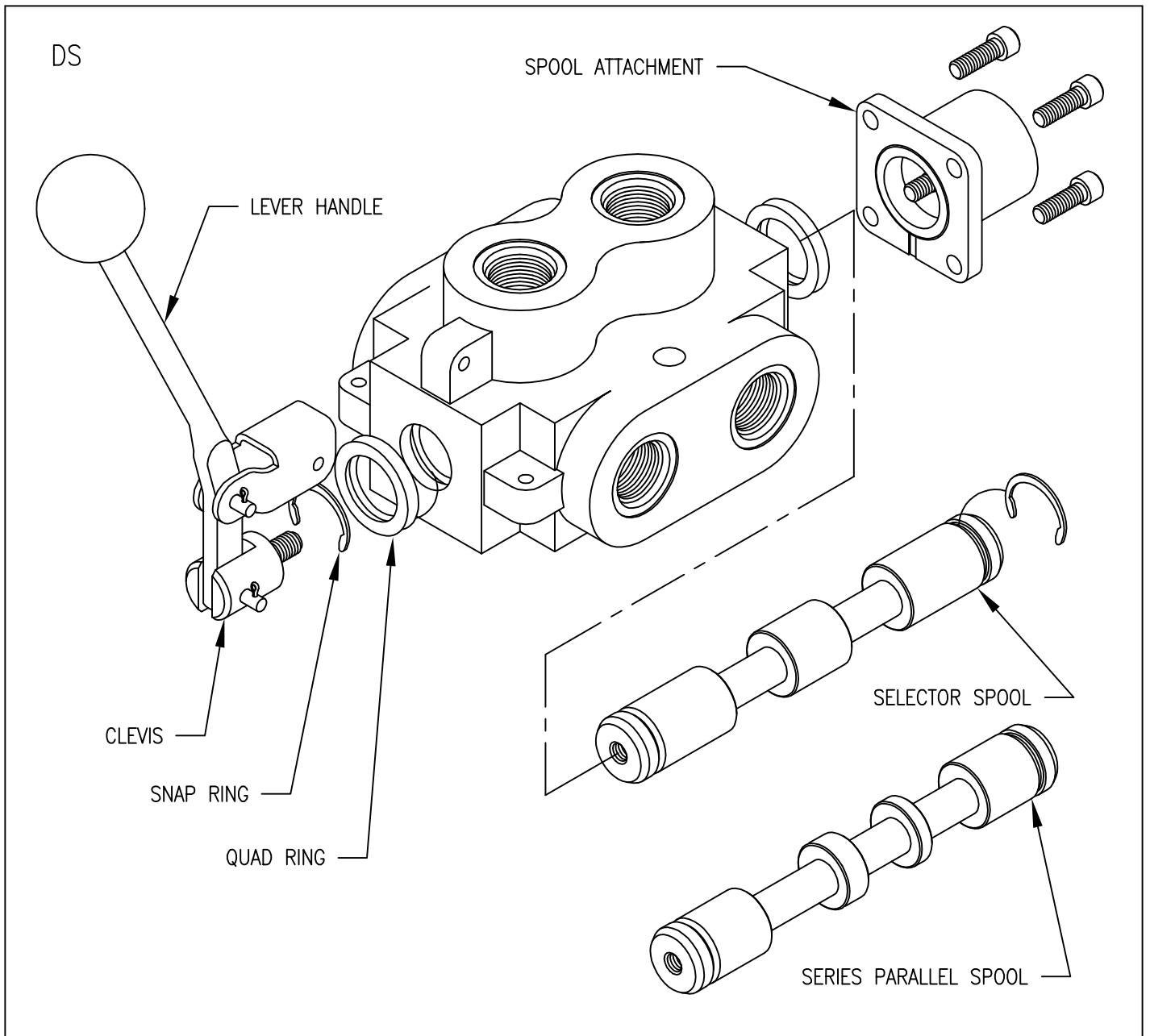
DS DOUBLE SELECTOR VALVE
